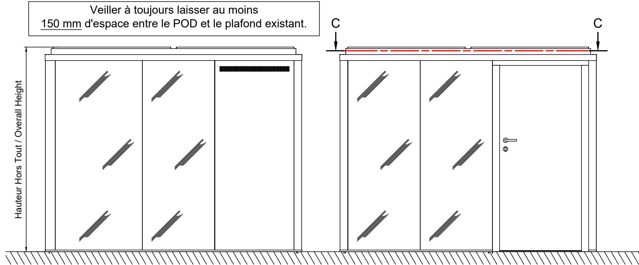
Coupe C-C
