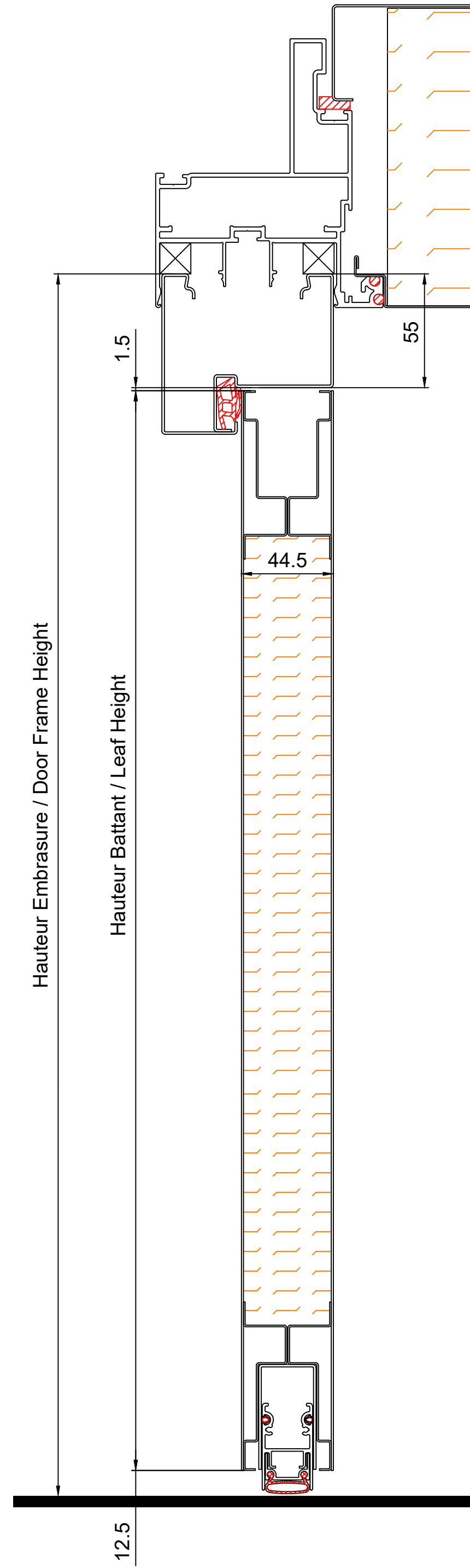
SECTION A-A
