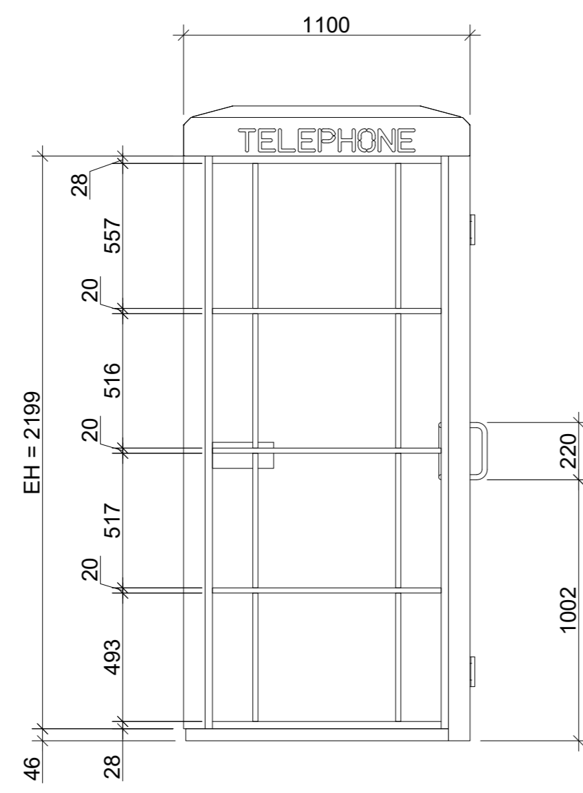
Ansicht B 1:20
