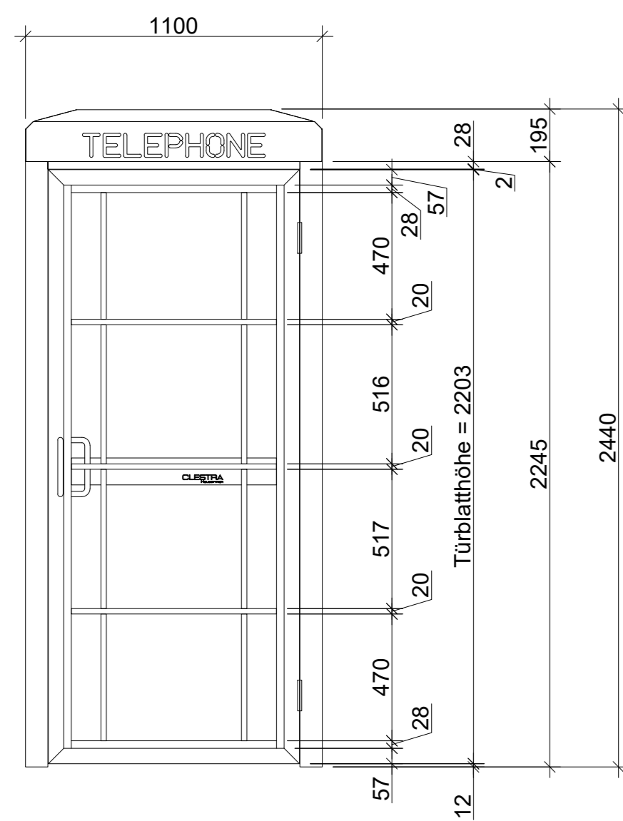
Ansicht A 1:20
