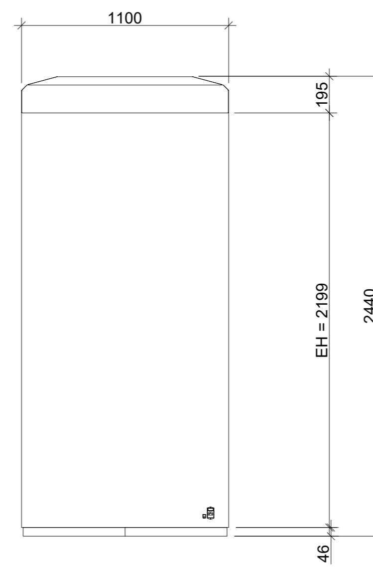
Ansicht C 1:20
