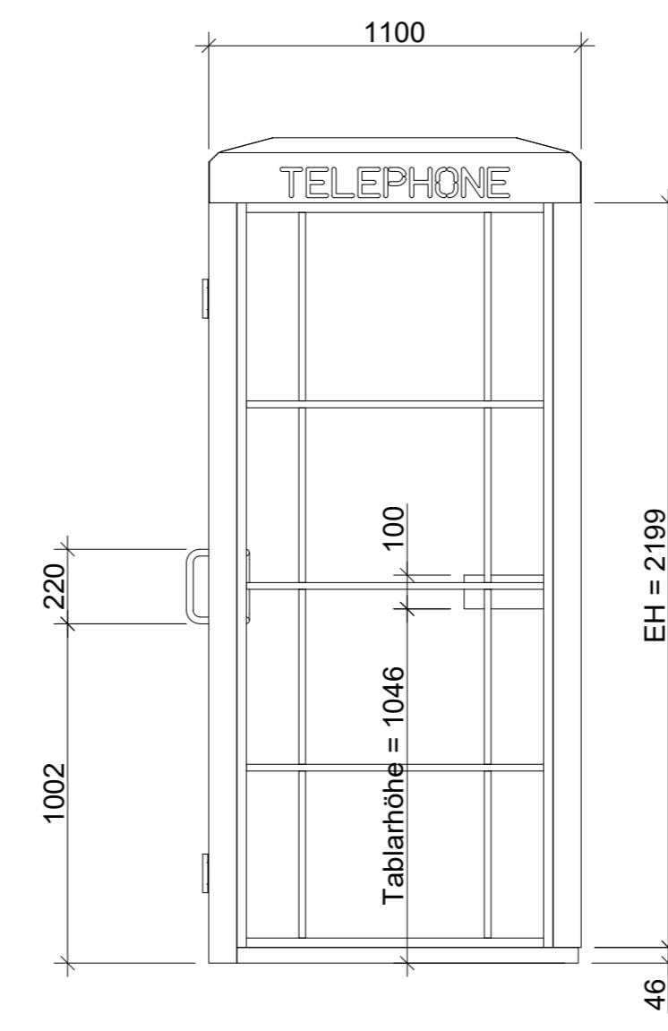
Ansicht D 1:20
